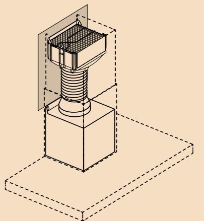
Exemple d'installation du module cleanAir Plus intégré*
